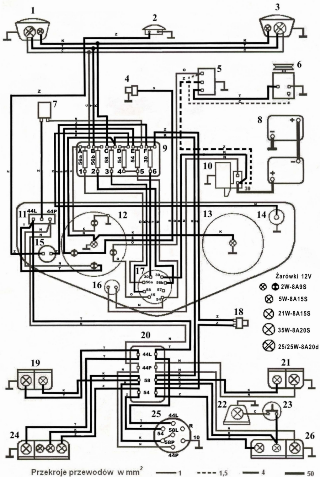
Schemat instalacji elektrycznej C-360 (prądnica)
